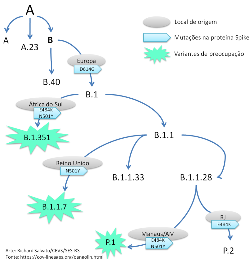
Figura 2: Representação da origem e características das principais linhagens do SARS-CoV-2 circulantes no Brasil
