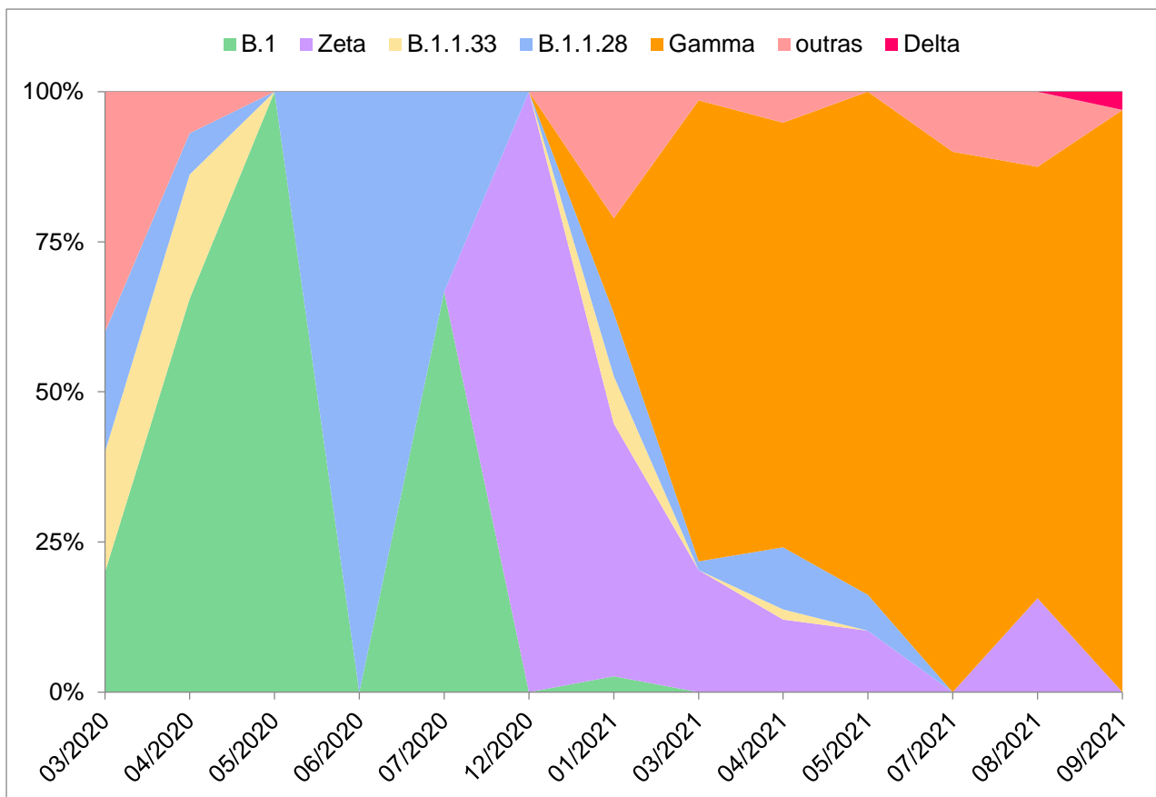
Gráfico 6 – Frequência das 05 linhagens mais frequentes em Sergipe
