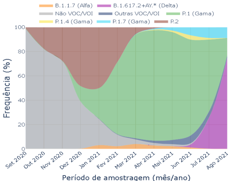
Figura 1: Principais linhagens em diferentes regiões do país (Fonte: Rede Genômica Fiocruz em 22/09/2021)
