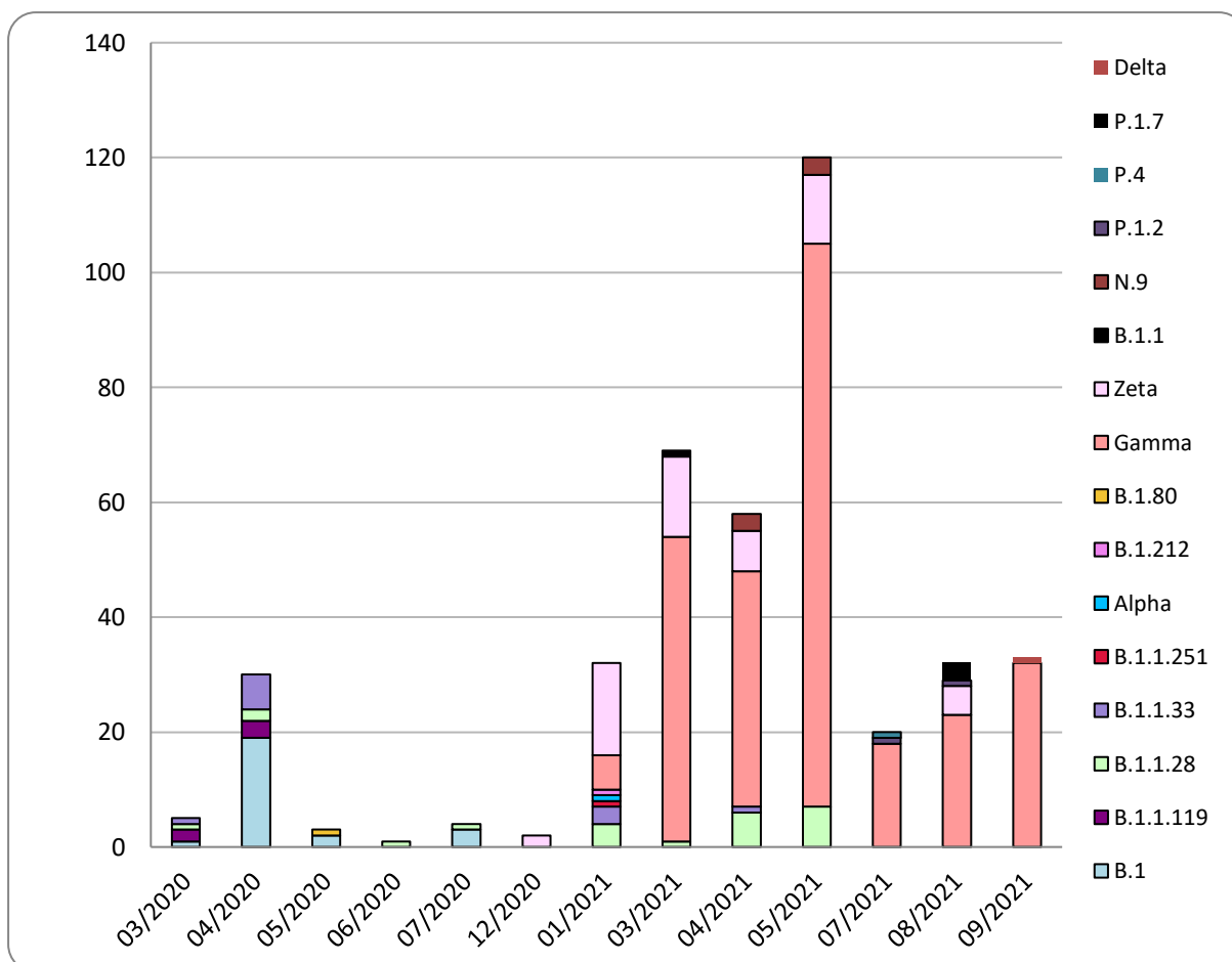
Gráfico 2 - Distribuição das diferentes linhagens nos diferentes meses de coleta das amostras
