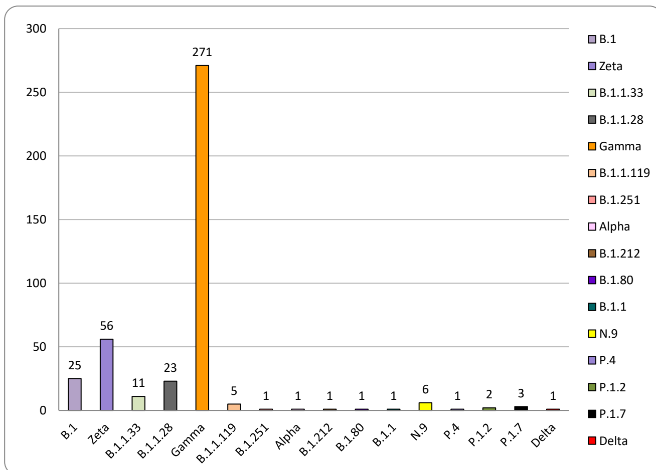
Gráfico 1- Proporção das diferentes linhagens do vírus SARS-CoV-2 circulantes no Estado
