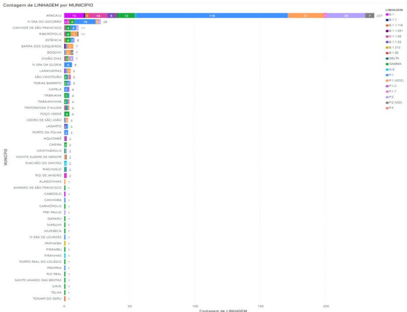
Gráfico 3 - Distribuição das diferentes linhagens nos municípios sergipanos
